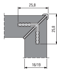
921 013 Profil für 16 mm 921 015 Profil für 19 mm
