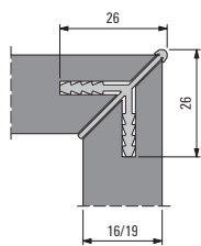
921 012 Profil für 16 mm 921 014 Profil für 19 mm
