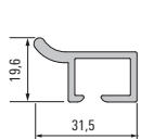
928 058 Linero function strip
