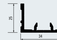
Aufsatzleiste Attachment rail 100008701
