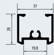
Rahmenprofil 19 oben / unten Frame profile 19 top / bottom 100008713
