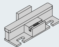
Glasschuh mit Glasauflage und Glasklotz Glass shoe with glass support and glazing block 100023709 100023881 100023708
