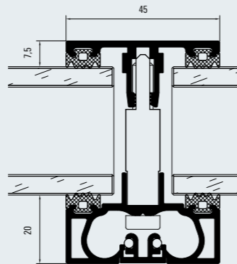
Horizontalschnitt Trägerprofil XL Horizontal section detail of load-bearing profile XL
