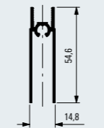
Rahmen unten Bottom frame 100008316
