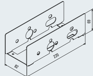
Schlosskasten für Türprofil Premium L-XL Lock case for premium door profile L-XL 100022604
