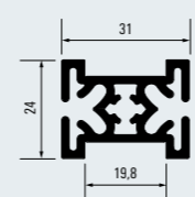
Sprossenprofil 19 Glazing bar profile 19 100008724
