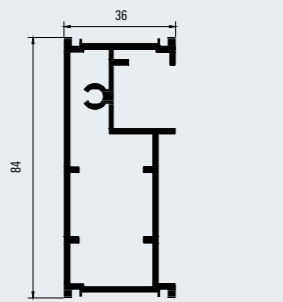
Türprofil unten Premium L-XL Premium bottom door profile L-XL 100022348
