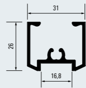
Rahmenprofil 16 oben / unten Frame profile 16 top / bottom 100008680
